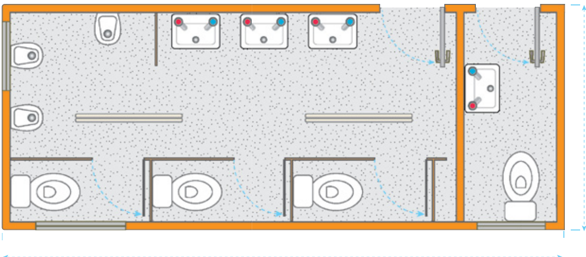
Toilet unit
